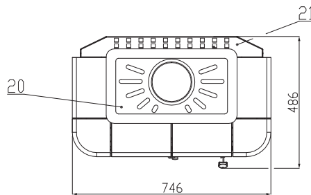
Rozmer kúreniska
