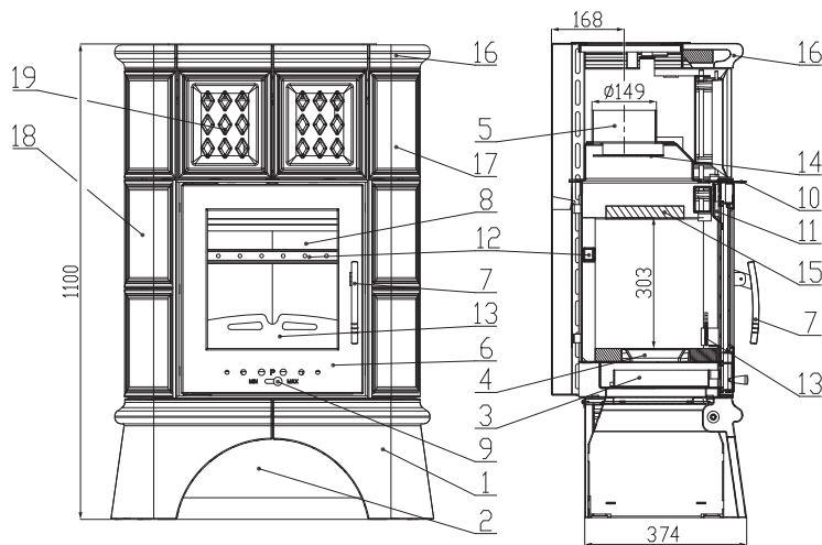
Rozmer kúreniska
