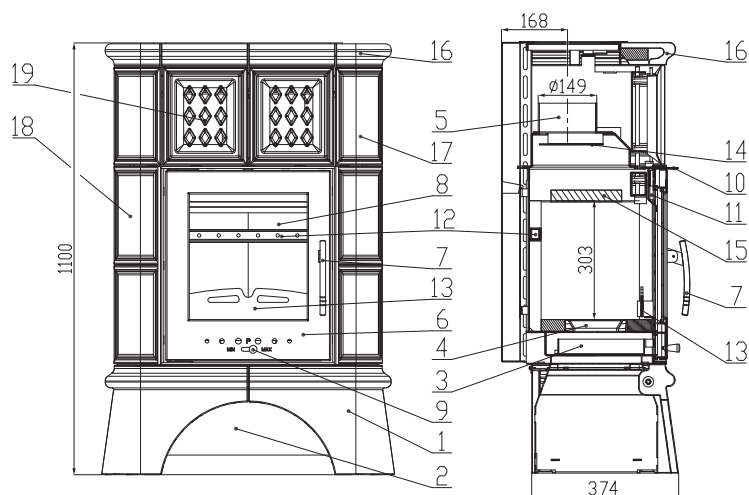
Rozměr topeniště
