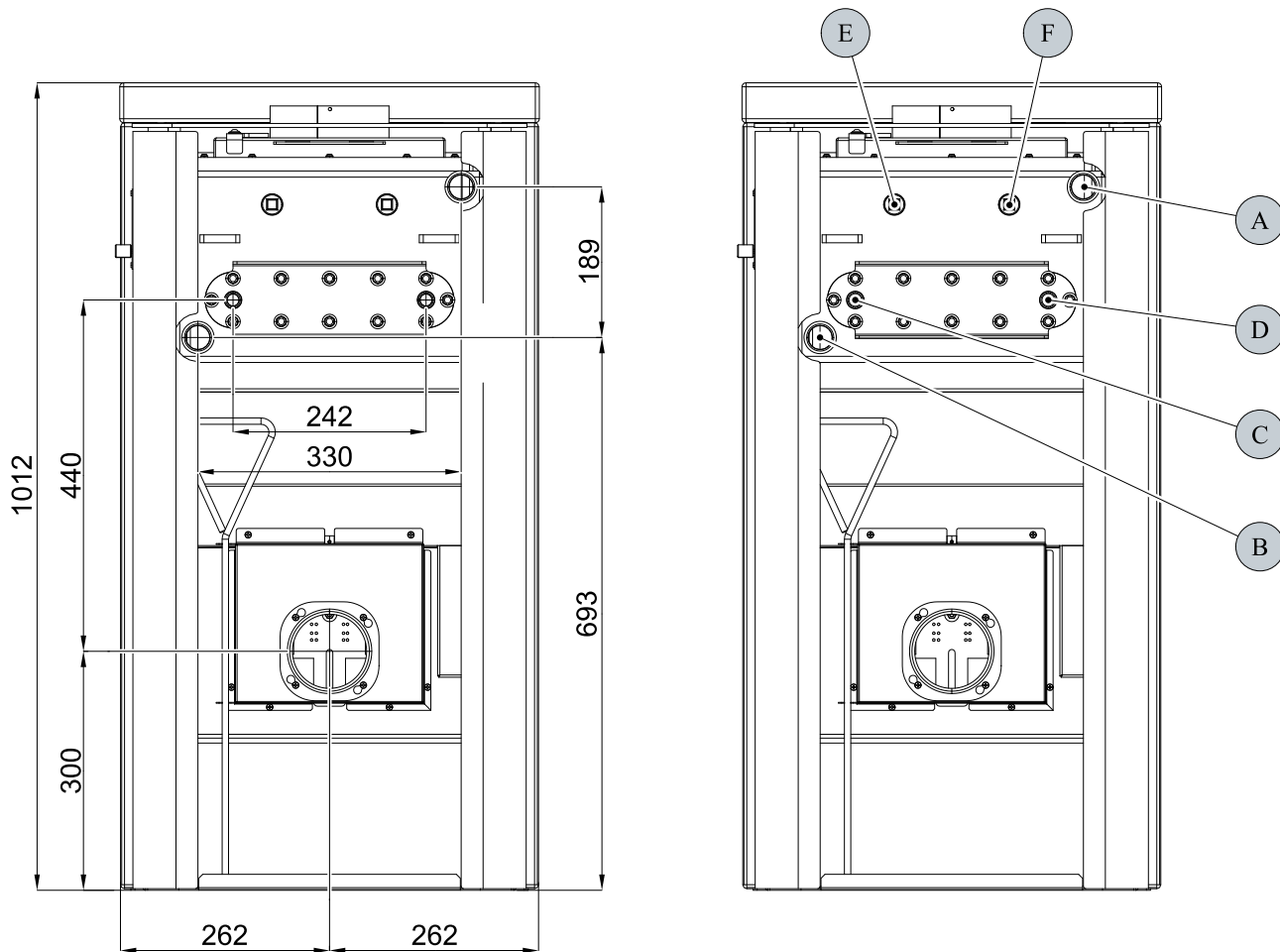
Rozměrové schéma
